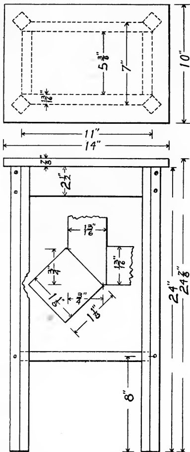
Fig. 196—Taboret
